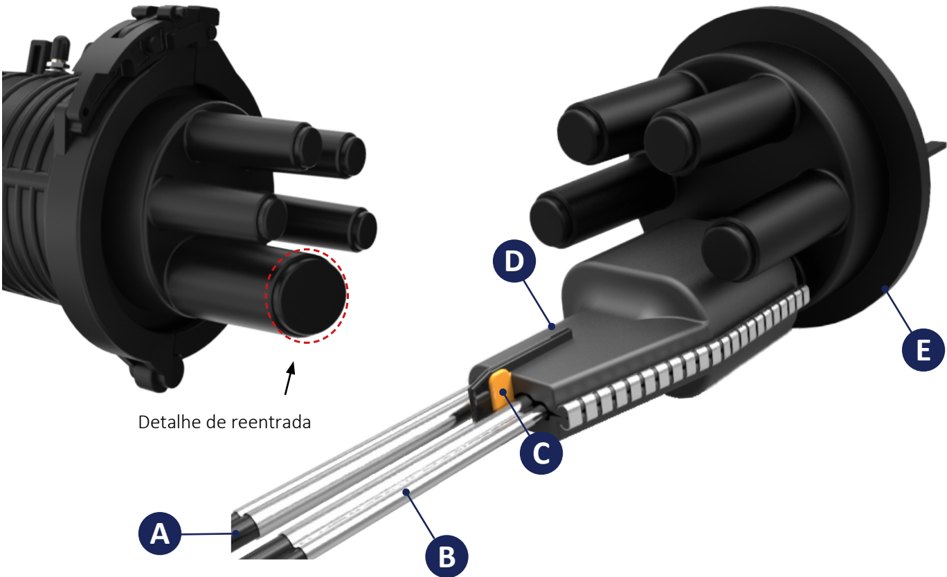
A. Cabos óptico; B. Fita de alumínio; C. Clipe metálico; D. Manta zipada; E. Base CEO.
